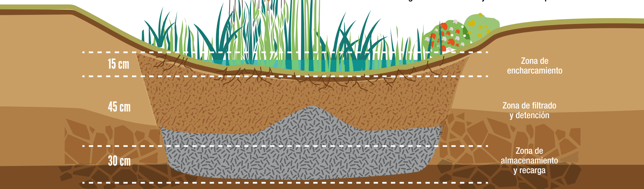
Figura 4. Corte de un jardín de lluvia típico
